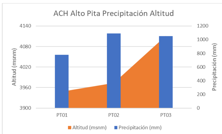
Figura 2. Precipitación media anual respecto a altitud de las estaciones en las microcuencas de monitoreo de impacto - ACHAP, la media de la estación PT02 no incluye el año 2018 ya que se encuentra incompleto.
