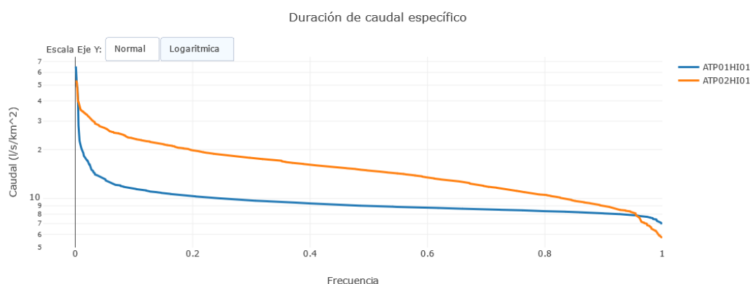
Figura 4. Curva de duración de caudales para la microcuenca de Tungurahua ATP01HI01 y Chamilco ATP02HI01
